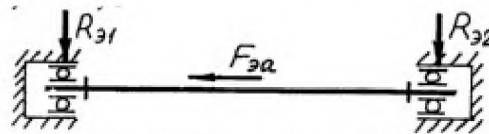
Рис 9.3 Расчетная схема нагружения шариковых подшипников
