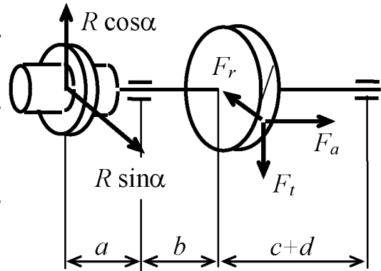
Рис. 8.2 Схема нагружения тихоходного вала редуктора
